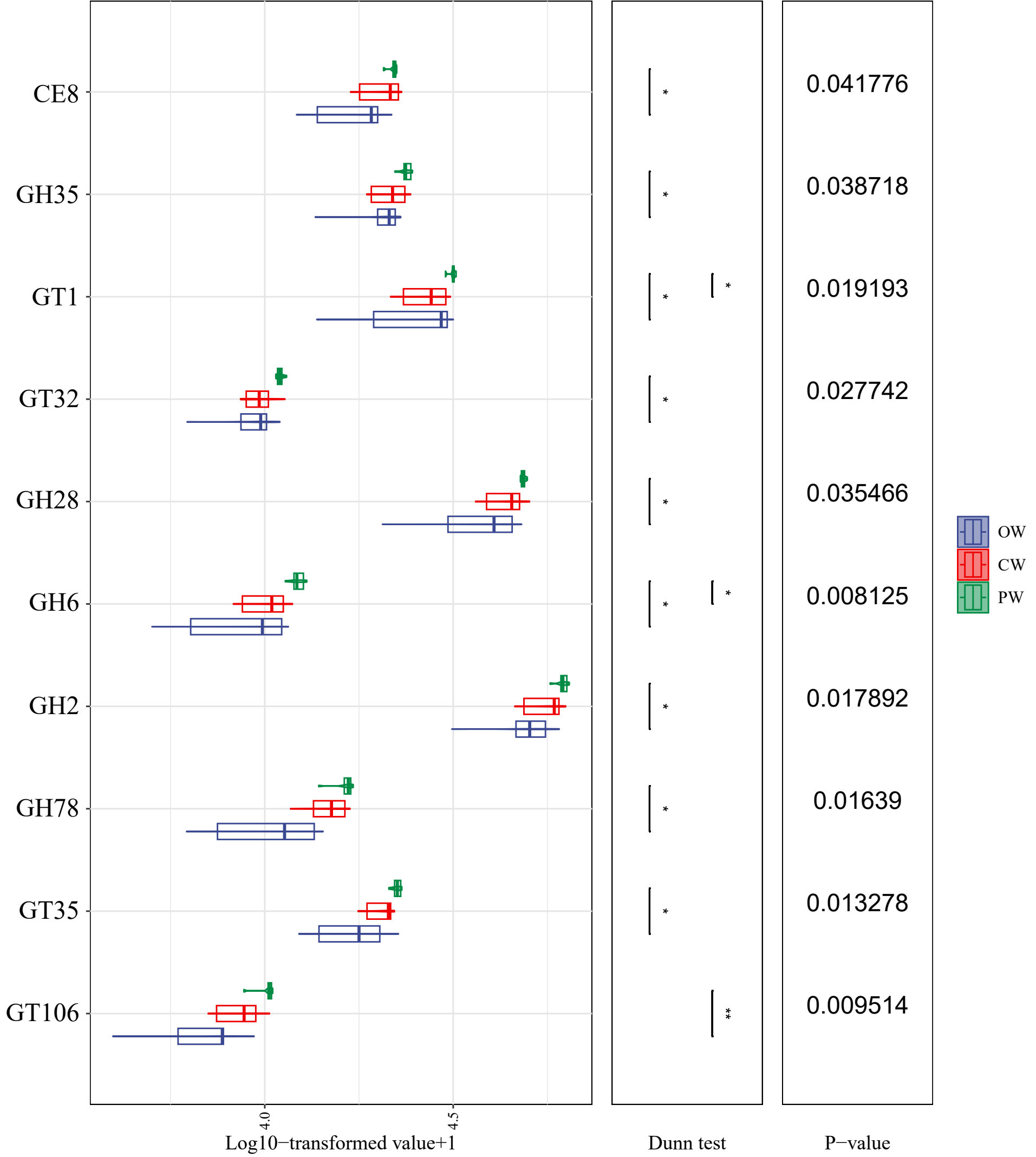
Kruskal–Wallis test
